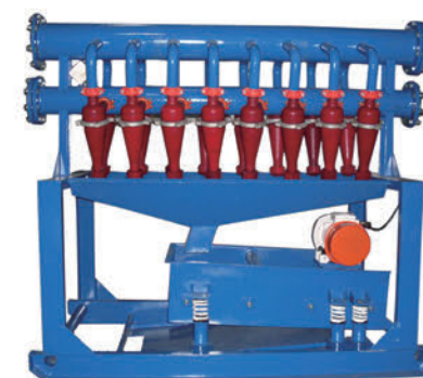
除泥器 Desilter
